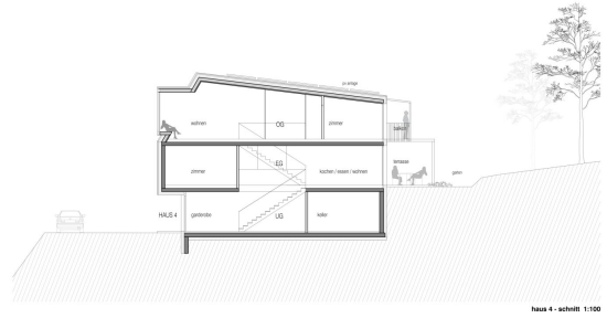
haus 4 - schnitt 1:100
