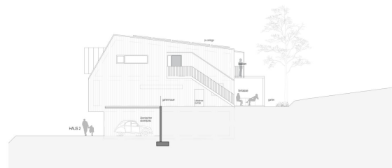
haus 2 - ansicht 1:100
