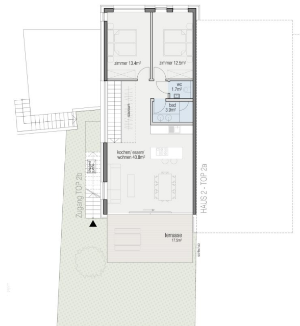
haus 2 - grundriss erdgeschoß 1:100
